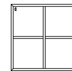
Art. CMP/55 Pensile libreria 4 vani cm. L59 P36 H59
