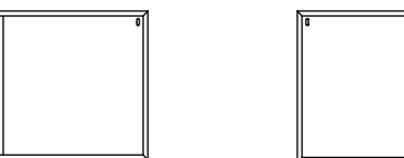
Art. CMP/22 Base 2 cestoni lisci cm. L177 P58 H32 Art. CMP/23 Base 2 cestoni lisci senza basamento cm. L177 P58 H29,5
