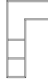
Art. CMP/49/SX Pensile libreria SX 3 vani ruotabile cm. L66,5 P36 H118 cm. L29,5 H88,5 angolo 37
